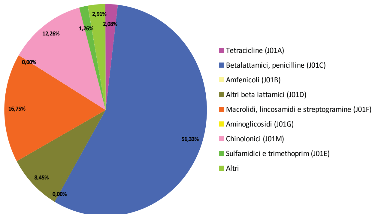
Figura 2.16 - Distribuzione del consumo di antibiotici per uso sistemico in Italia in comunità 2014.
