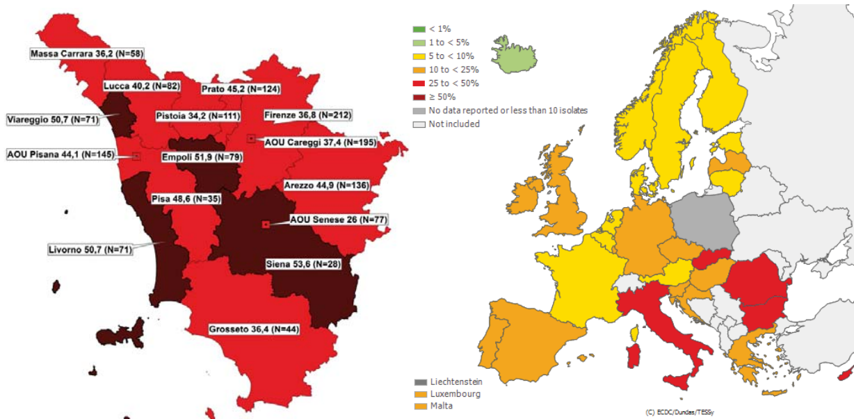
Figura 3.9 - E. coli : percentuale (%) di isolati resistenti a Cefalosporine di III generazione nei territori delle aziende sanitarie toscane (Toscana, 2014) e nei paesi europei (2014).
