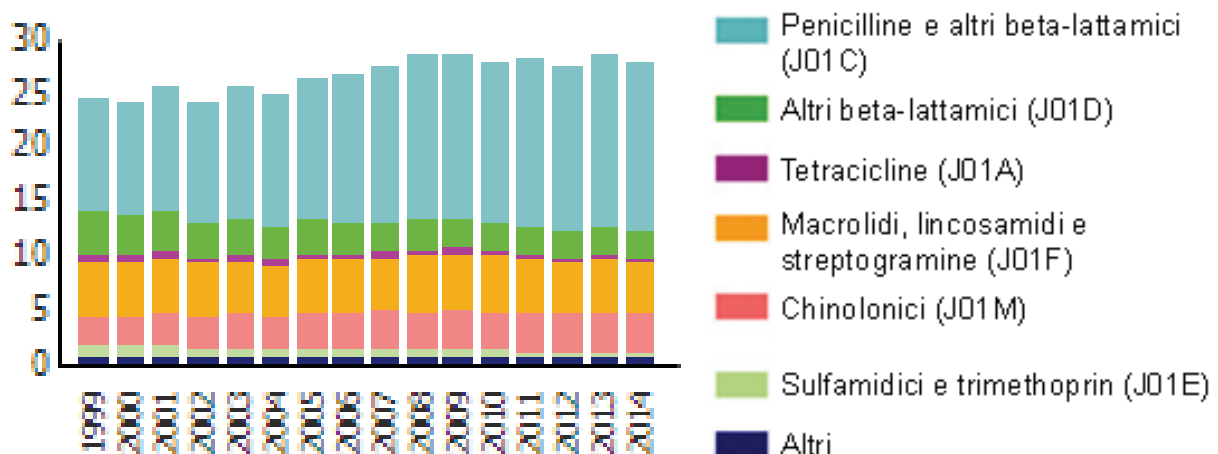
Figura 2.15 - Andamento del consumo territoriale di antibiotici ad uso sistemico in Italia per classi e anno (DDD/1.000 abitanti/die).
