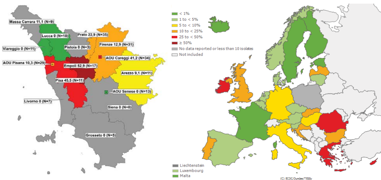
Figura 3.5 - E. faecium : percentuale (%) di isolati Vancomicino-resistenti (VRE), nei territori delle aziende sanitarie toscane (Toscana 2014) e nei paesi europei (2014).
