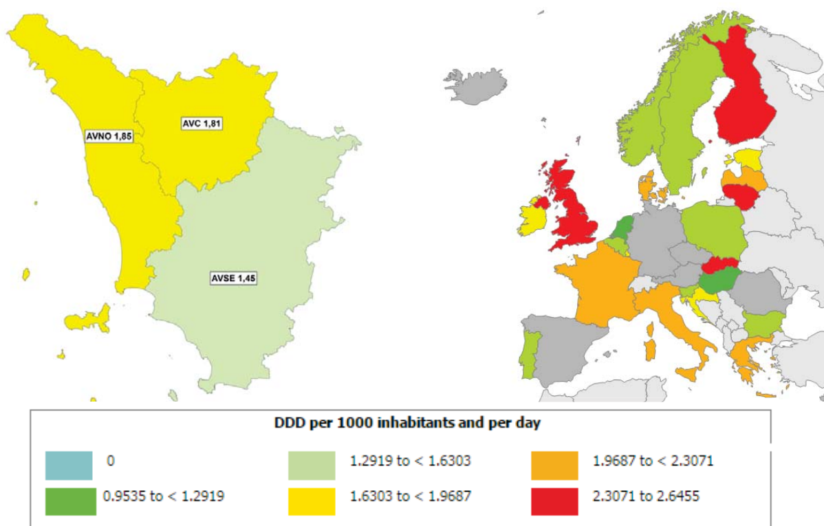
Figura 2.9 - Distribuzione percentuale del consumo (DDD/1.000 abitanti/die) di beta-lattamici, penicilline (J01C) per Area Vasta di residenza (Toscana 2014) e paesi europei (2014).
