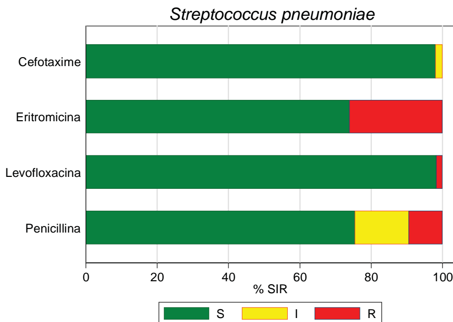
Figura 3.6 - Profili di sensibilità agli antibiotici saggiati su isolati di S. pneumoniae . Toscana 2014 (S: sensibile; I: intermedio; R: resistente).
