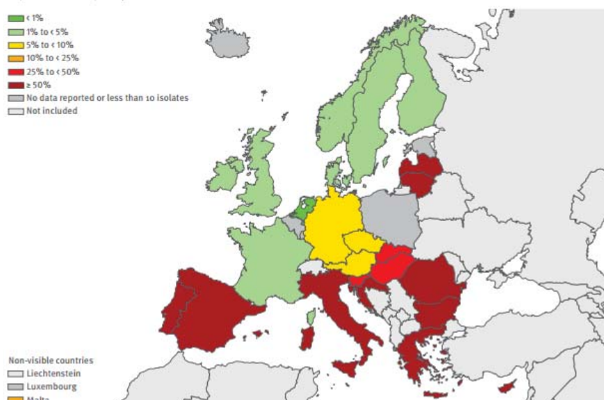
Figura 3.21 - Acinetobacter spp.: percentuale (%) di isolati resistenti carbapenemi nei paesi europei (2014) - valore medio toscano: 80,5%; valore medio italiano: 70,9%.
