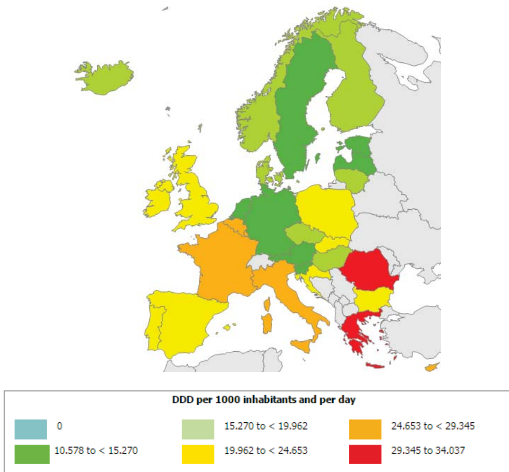
Figura 2.13 - Consumo di antibiotici a uso sistemico (J01) sul territorio in Europa (dati ESAC, anno 2014).
