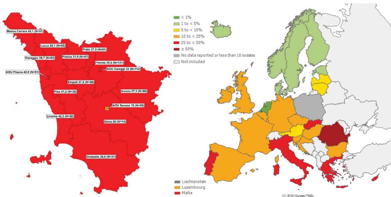
Figura 3.2 - S. aureus : percentuale (%) di isolati meticillino-resistenti (MRSA) nei territori delle aziende sanitarie toscane (Toscana 2014) e nei paesi europei (2014).
