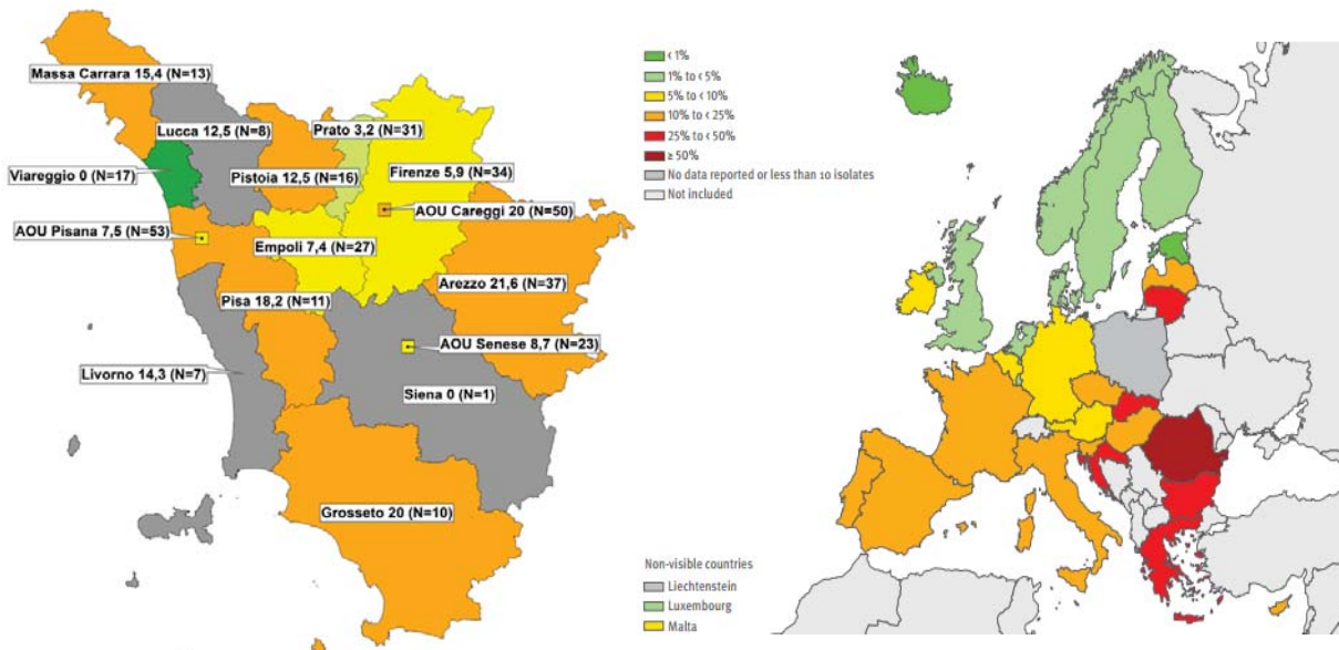
Figura 3.19 - P. aeruginosa : percentuale (%) di isolati resistenti ad almeno 3 tra Piperacillina/Tazobactam, Ceftazidime, fluorochinoloni, aminoglicosidi e carbapenemi nei territori delle aziende sanitarie toscane (Toscana, 2014) e nei paesi europei (2014).
