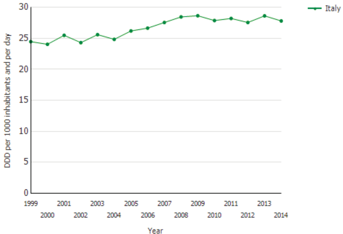
Figura 2.15 - Andamento del consumo territoriale di antibiotici ad uso sistemico in Italia per classi e anno (DDD/1.000 abitanti/die).
