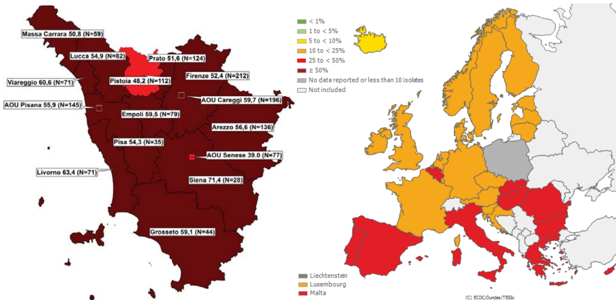
Figura 3.8 - E. coli : percentuale (%) di isolati fluorochinoloni-resistenti nei territori delle aziende sanitarie toscane (Toscana, 2014) e nei paesi europei (2014).
