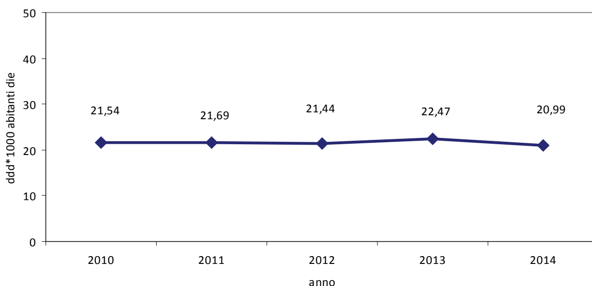
Figura 2.17 - Consumo territoriale di antibiotici per uso sistemico (J01) in Toscana. Anni 2010-2014.
