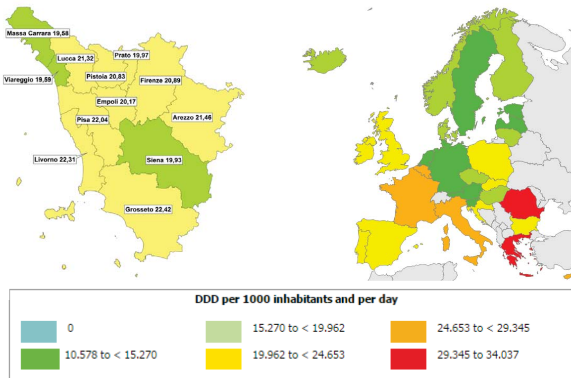
Figura 2.19 - Distribuzione percentuale del consumo (DDD/1.000 abitanti/die) di antibiotici ad uso sistemico (J01) per ASL di residenza (Toscana 2014) e paesi europei (2014).
