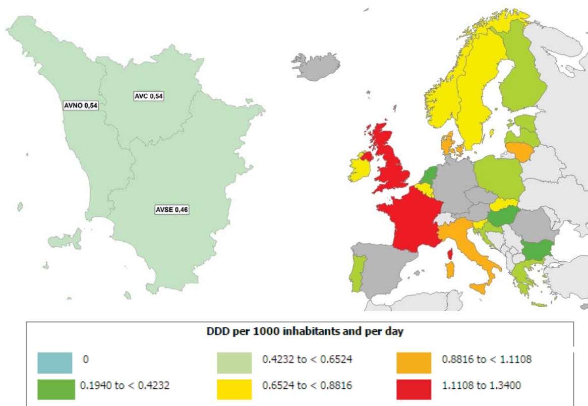
Figura 2.9 - Distribuzione percentuale del consumo (DDD/1.000 abitanti/die) di beta-lattamici, penicilline (J01C) per Area Vasta di residenza (Toscana 2014) e paesi europei (2014).
