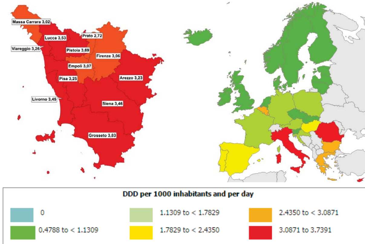
Figura 2.21 - Distribuzione percentuale del consumo (DDD/1.000 abitanti/die) di chinoloni (J01M) per ASL di residenza (Toscana 2014) e paesi europei (2014).
