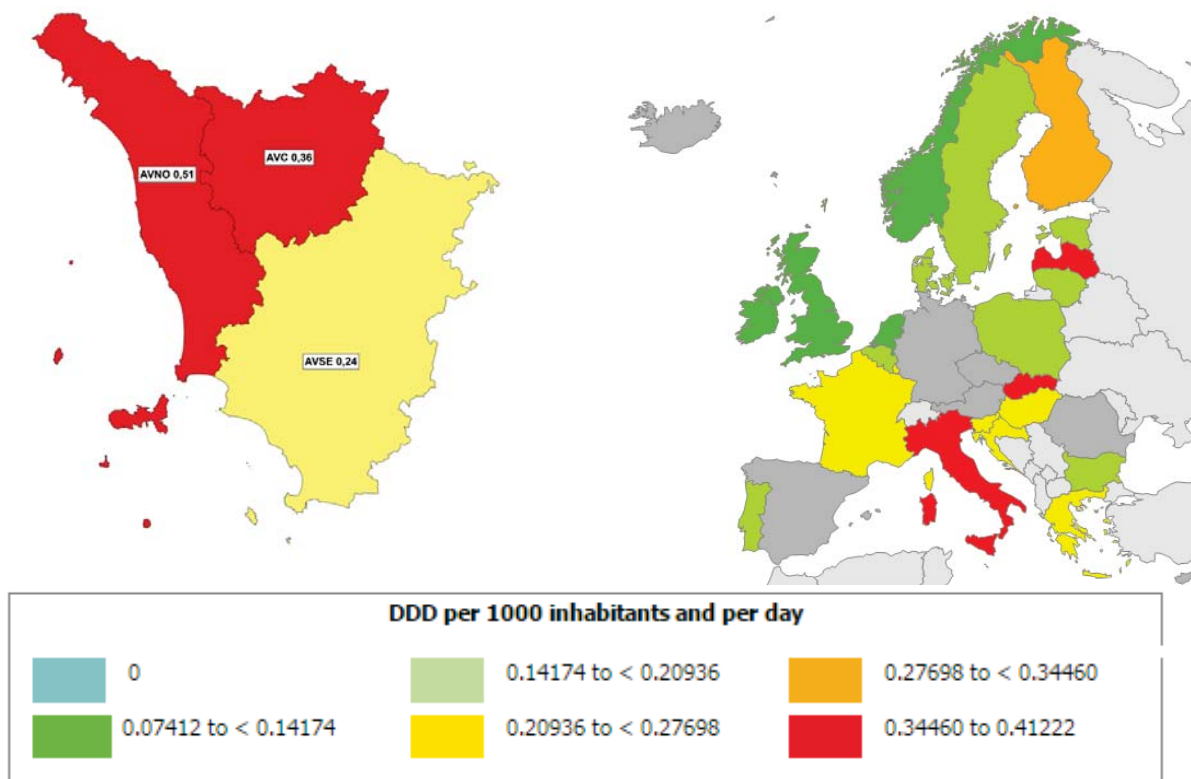
Figura 2.12 - Distribuzione percentuale del consumo (DDD/1.000 abitanti/die) di chinoloni (J01M) per Area Vasta di residenza (Toscana 2014) e paesi europei (2014).
