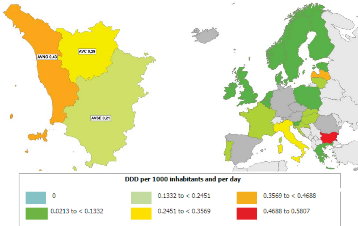
Figura 2.11 - Distribuzione percentuale del consumo (DDD/1.000 abitanti/die) di carbapenemi (J01DH) per Area Vasta di residenza (Toscana 2014) e paesi europei (2014).
